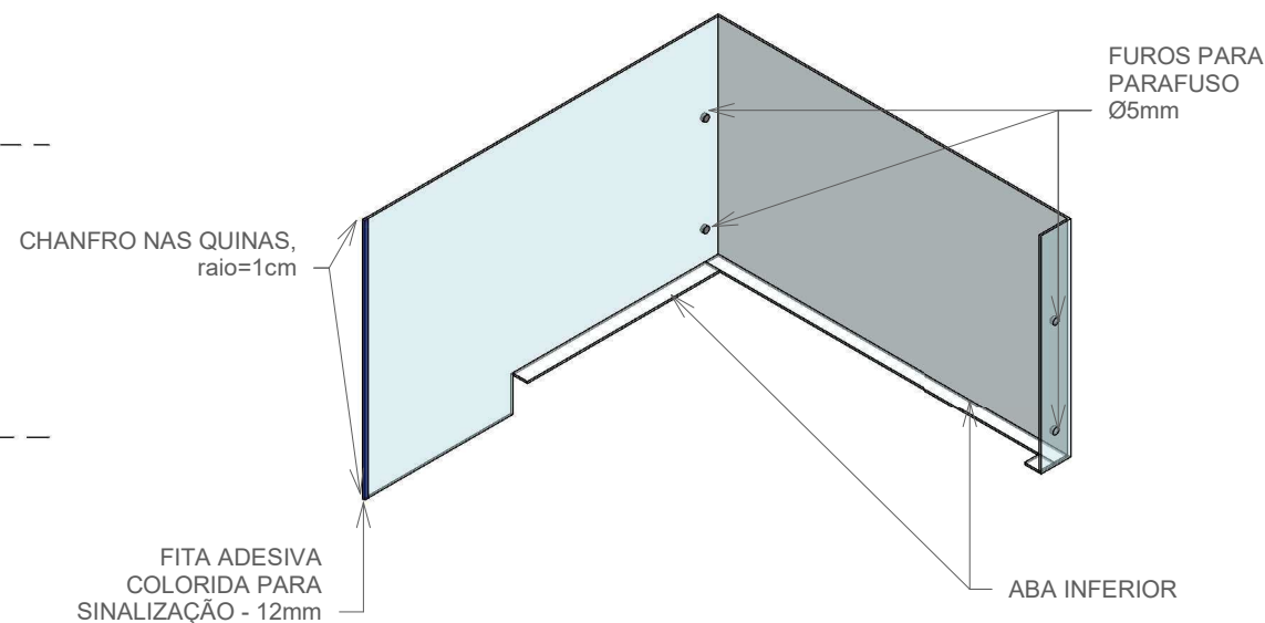
4 ISOMÉTRICA
