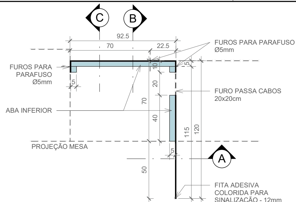
1 PLANTA 1 : 20
