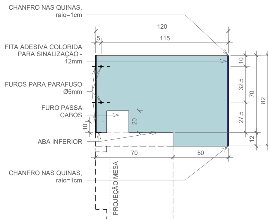
3 CORTE B 1 : 20
