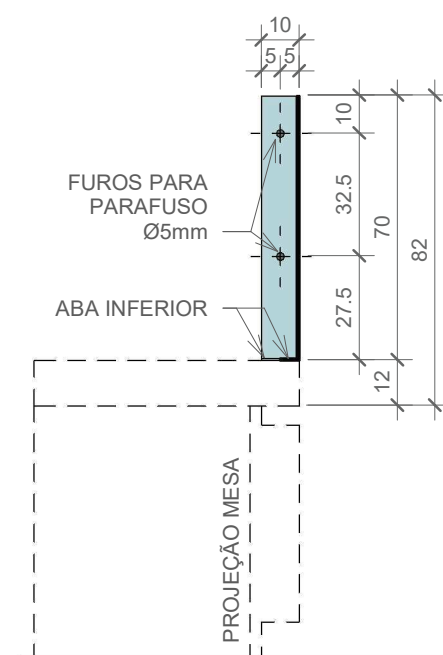
4 CORTE C 1 : 20
