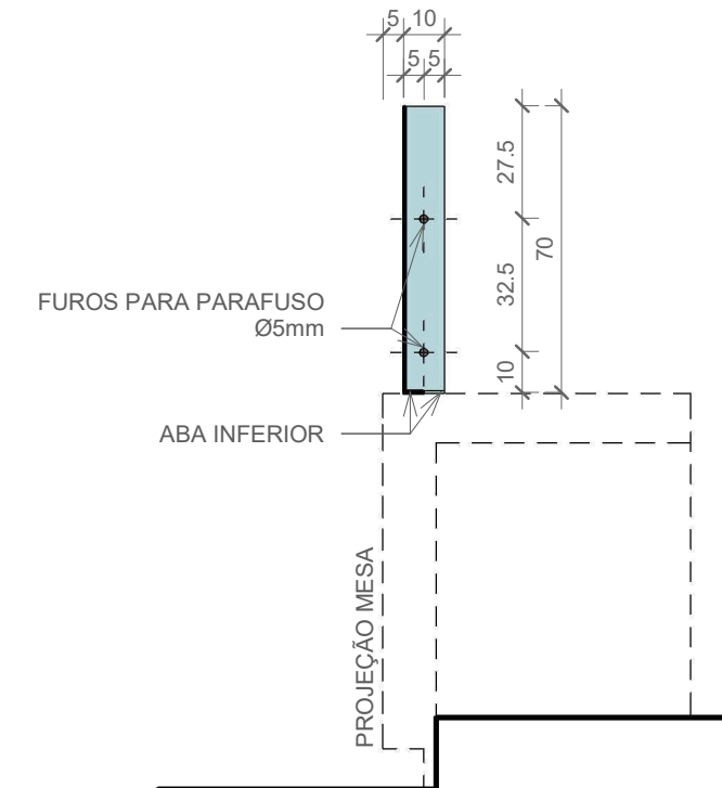
6 CORTE C 1 : 20
