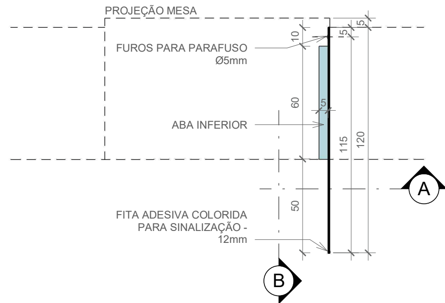
1 PLANTA 1 : 20
