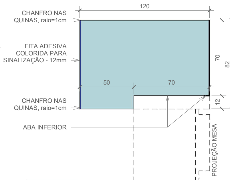
3 CORTE B 1 : 20
