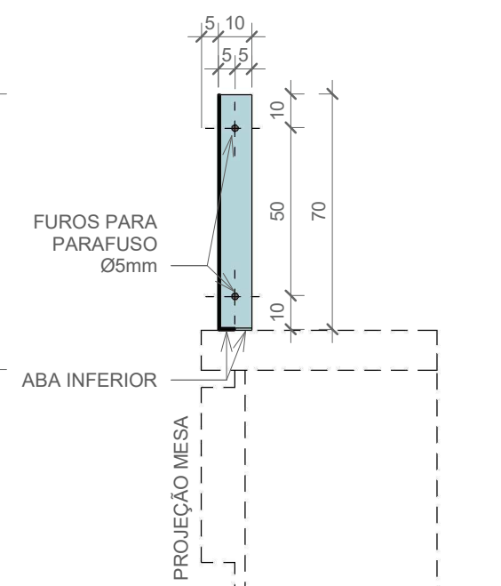
4 CORTE C 1 : 20
