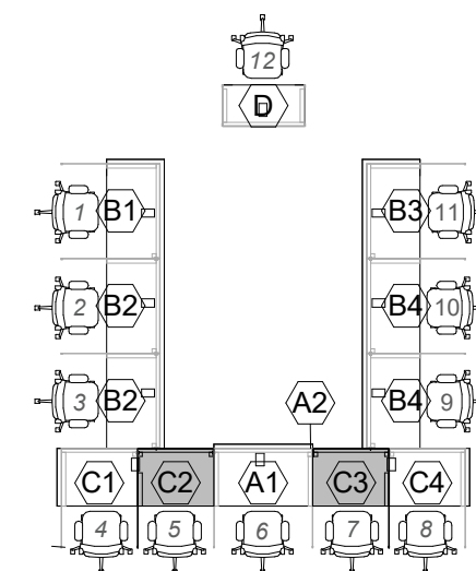
8 PLANTA CHAVE - C2 e C3 1 : 100
