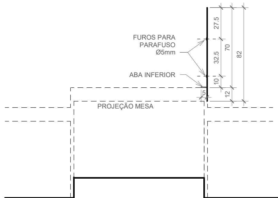
2 CORTE A 1 : 20
