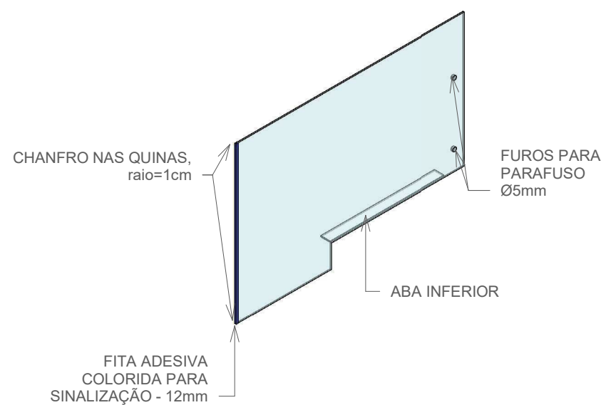
4 ISOMÉTRICA
