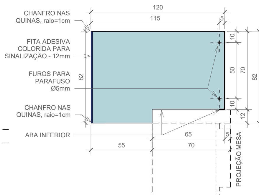
3 CORTE B 1 : 20
