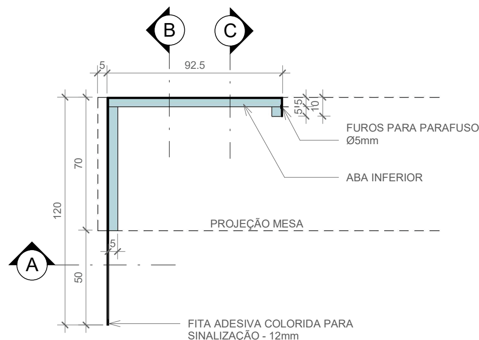
1 PLANTA 1 : 20
