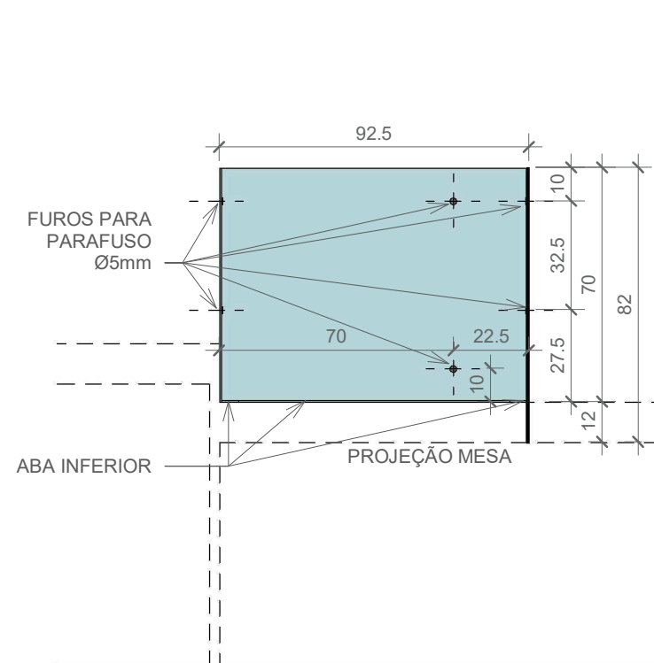
2 CORTE A 1 : 20
