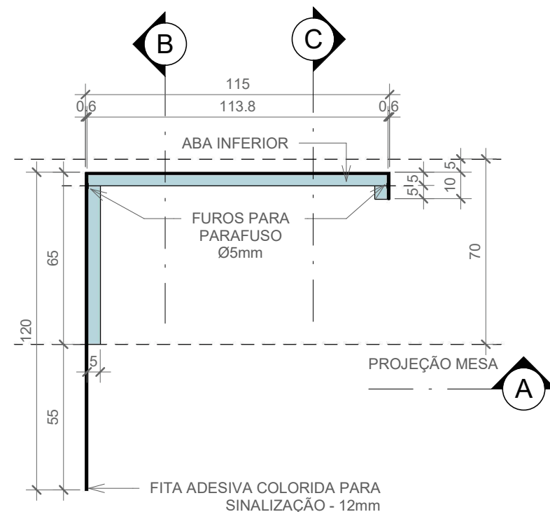
1 PLANTA 1 : 20
