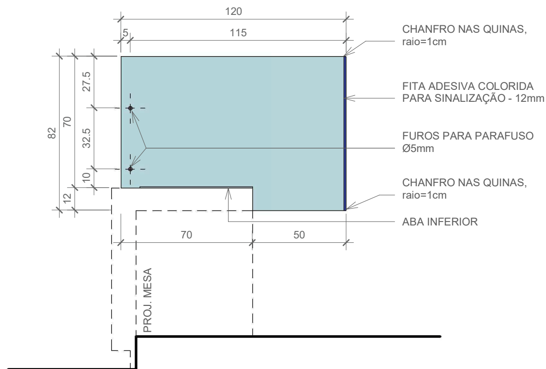
3 CORTE B 1 : 20
