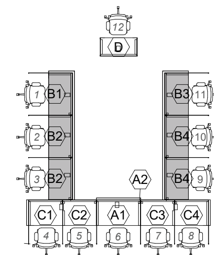
10 PLANTA CHAVE - MODELO B 1 : 100
