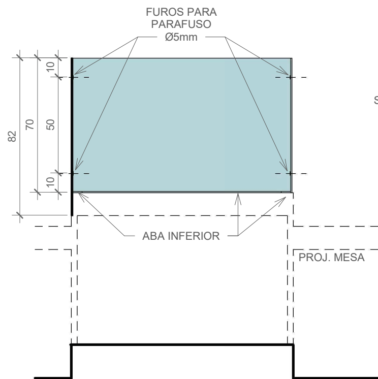
2 CORTE A 1 : 20
