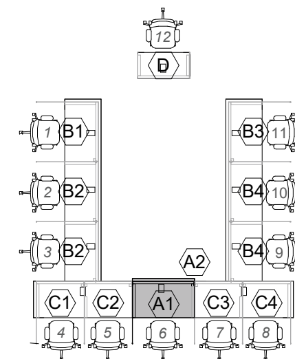
5 PLANTA CHAVE - MODELO A1 1 : 100
