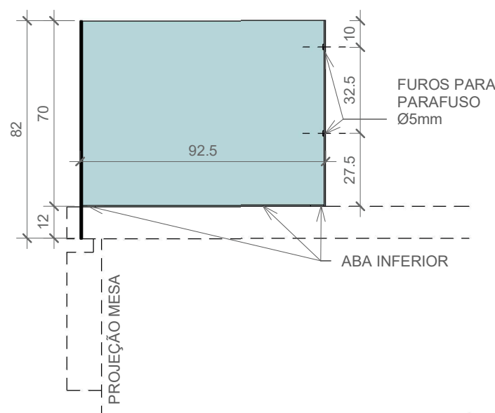
2 CORTE A 1 : 20
