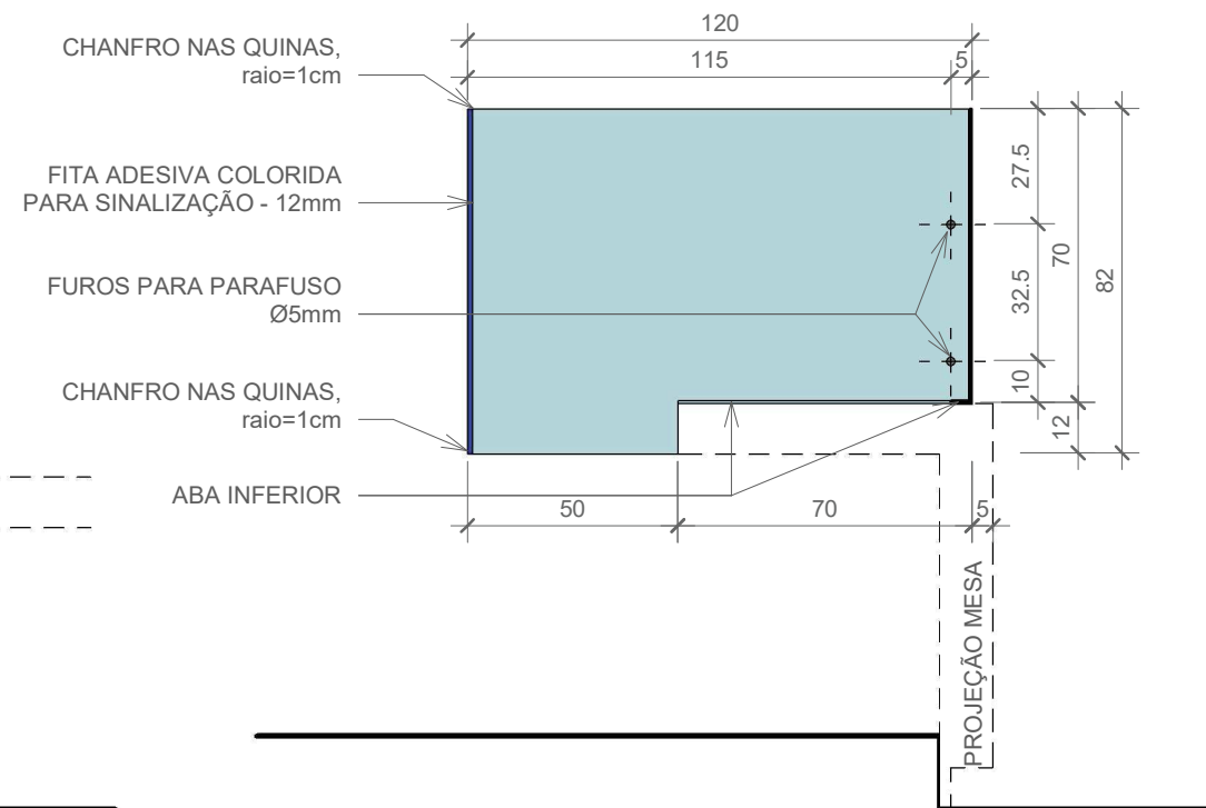
3 CORTE B 1 : 20
