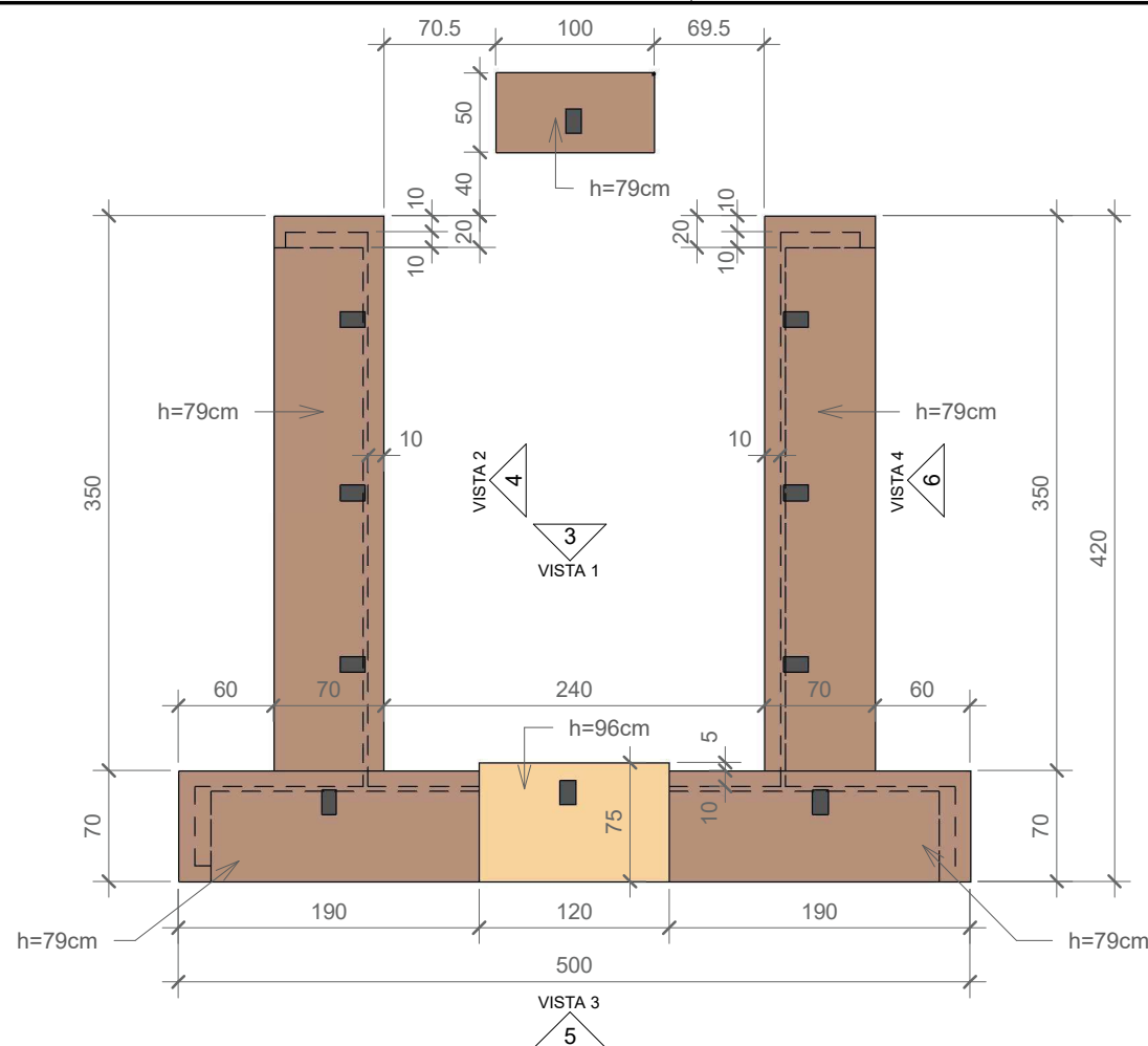
1 Planta - mesa plenário
