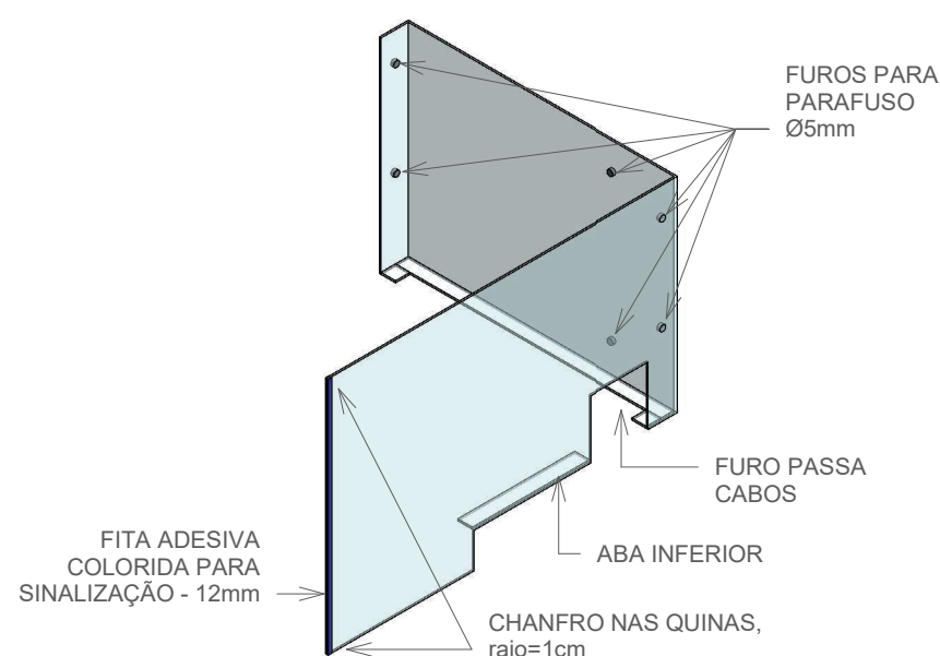
5 ISOMÉTRICA
