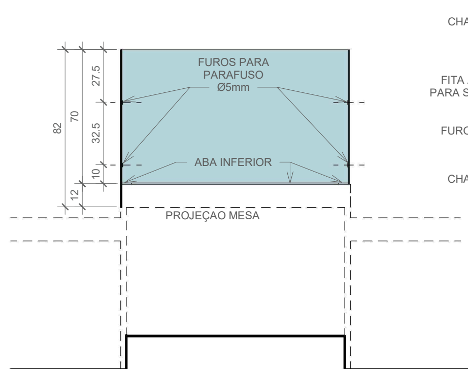
2 CORTE A 1 : 20
