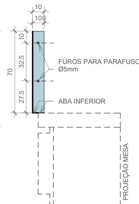
4 CORTE C 1 : 20
